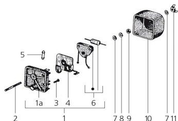
Vespa 50-125 PV/ET3/S/SS
